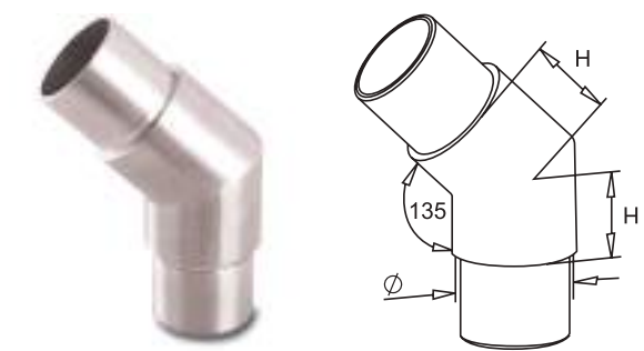
45° ELBOW
